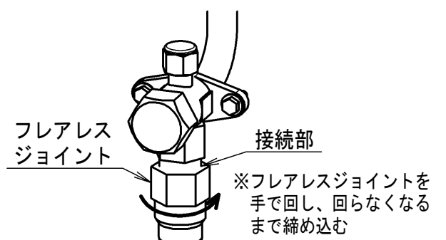
図8 室外ユニット接続イメージ
